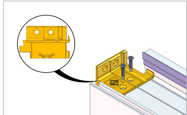
7. Verbinder am vorgebohrten Aufbauprofil mit 2 Schrauben M3,9 x 19 mm (141.003.019.000) verschrauben.
