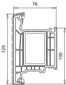
105.401 außen öffnend Verstärkung 113.011, 113.011.5 vorgefräst
