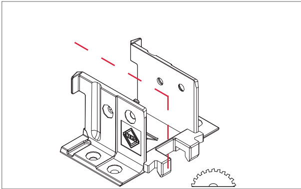
6. Verbinder 106.424 halbieren.
