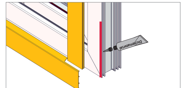
4. Bevor die Aluminium-Vorsatzblenden aufgeklipst werden, muss das Element seitlich (L+R) im markierten Bereich (150 mm) mit geeignetem Dichtmaterial abgedichtet werden.
