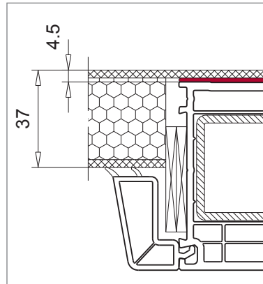
Außendeckschicht 4,5 mm inkl. Spalt für Kleber Spaltmaß Dichtung 3,5 mm
