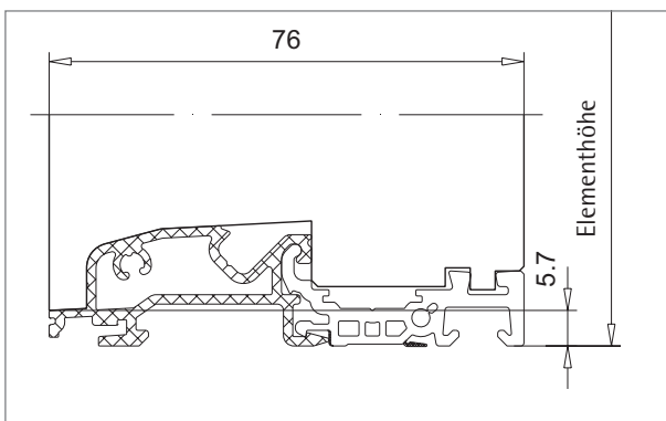
Fräsezeichnung für die Werkzeugbestellung
