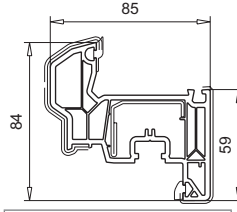
103.382 halbflächenversetzt Verstärkung 113.292, 113.294.2, 113.295, 113.394.2
