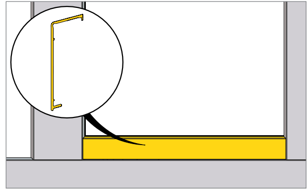
6. Aluminium-Vorsatzblende auf Länge schneiden, siehe ab Seite 6.86.
