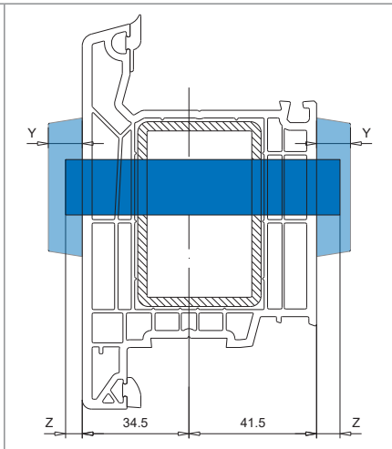
Flügel außen öffnend
