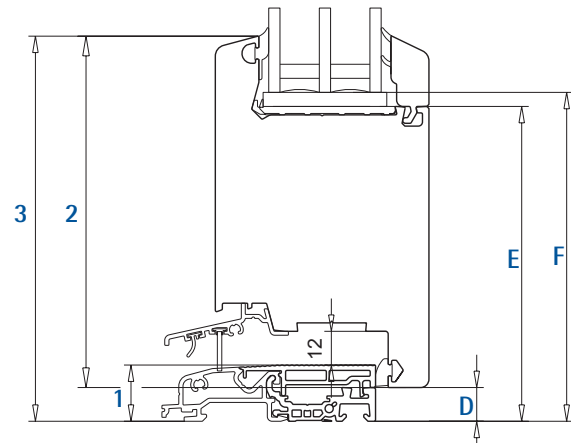
Bodenschwelle mit Flügel
