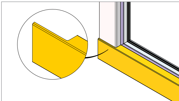
1. Horizontale Aluminium-Vorsatzblenden auf Länge schneiden, siehe ab Seite 6.86. Beidseitig stanzen, siehe Seite 6.48.
