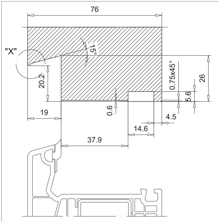
Fräszzeichnung für die Werkzeugbestellung AD
