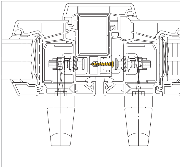
Stulpprofil 102.356 mit 2 Griffoliven (benötigt spezielle Schließbleche)
