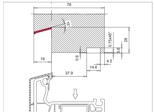
3. Für Aluminium-Vorsatzblenden muss die Standardfräsung angepasst werden (rot).
