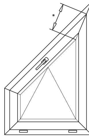
Kippfenster mit spitzem Winkel * Max. Schweißspiegelänge beachten!
