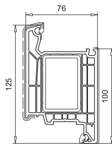
105.400 Verstärkung 113.011, 113.011.5 vorgefräst
