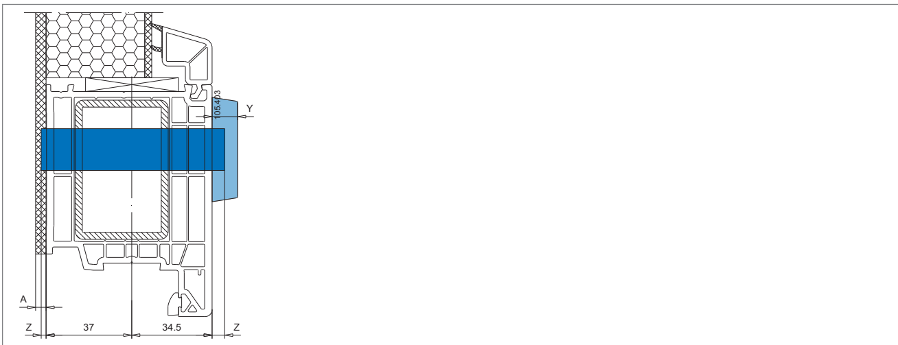
Flügel innen öffnend mit flügelüberdeckender Füllung: Profilzylinderlänge ist abhängig von der Außendeckschicht „A“ (im Beispiel mit 4,5 mm), siehe auch Seite 6.26
