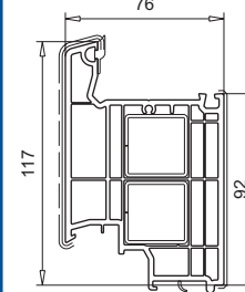
105.402 Aufbauprofil Verstärkung 113.025
