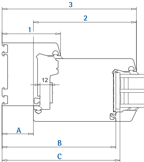
Rahmen-Flügel-Kombination
