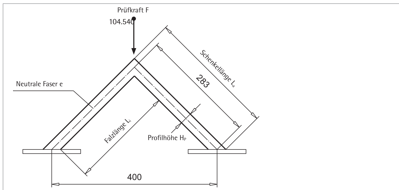
Prinzipische Skizze des Prüfaufbaus
