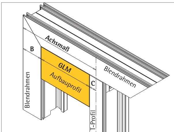
2. Aufbauprofil auf Länge schneiden für: Verbindung mit Verbinder = GLM. Maße für Blendrahmen und T-Profile, siehe Kapitel 4 Abzugsmaße.
