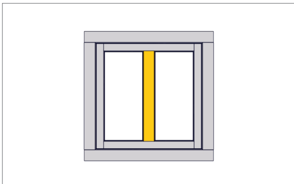
3. Aluminium-Vorsatzblenden für Flügelprosse am vorgefertigten Element positionieren und aufklipsen.
