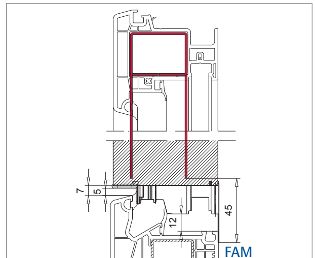
2. Verstärkung auf Länge schneiden (FAM - 90 mm) und im Profil einsetzen.
