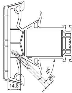
Vorkammerbelüftung T-Profil als Flügelprosse oben
