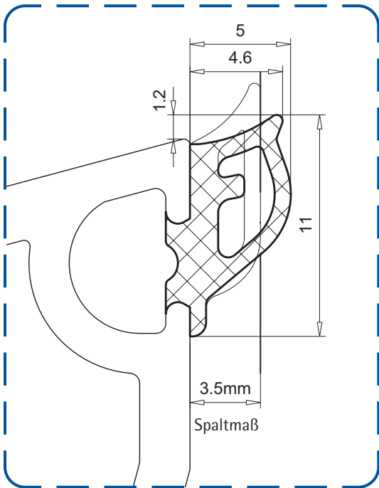
Blendrahmendichtungen 112.424 und 112.494
