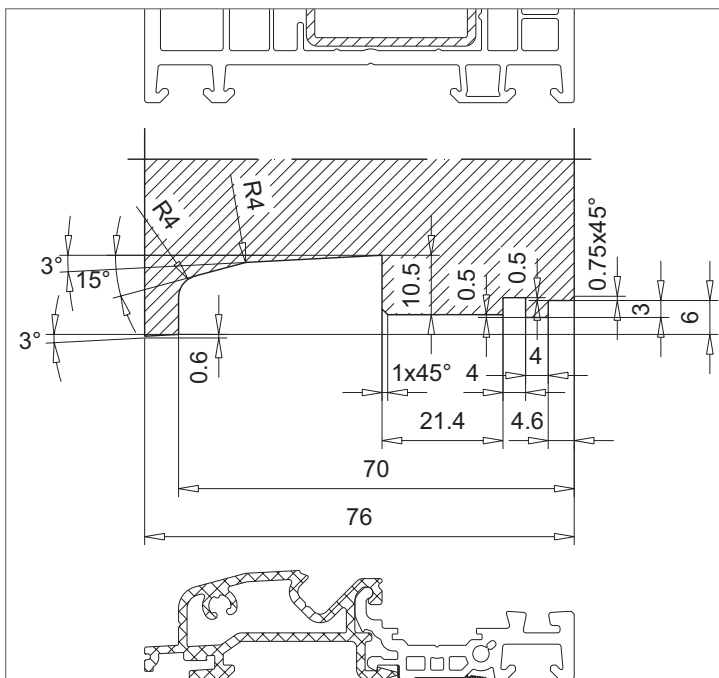
Fräsezeichnung für die Werkzeugbestellung
