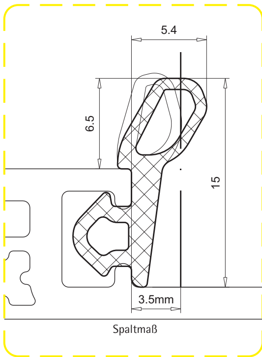
Mitteldichtungen 112.422
