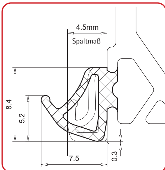
Flügelüberschlagdichtungen 112.496 und 112.354
