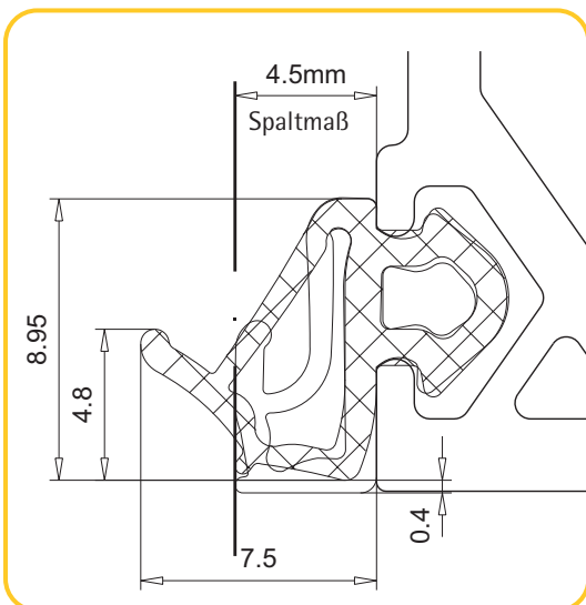
Flügelüberschlagdichtung 112.254
