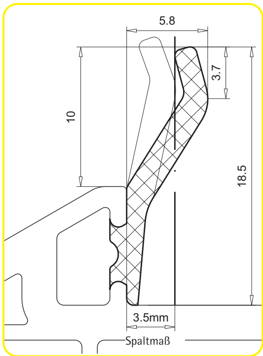
Mitteldichtungen 112.492 und 112.498
