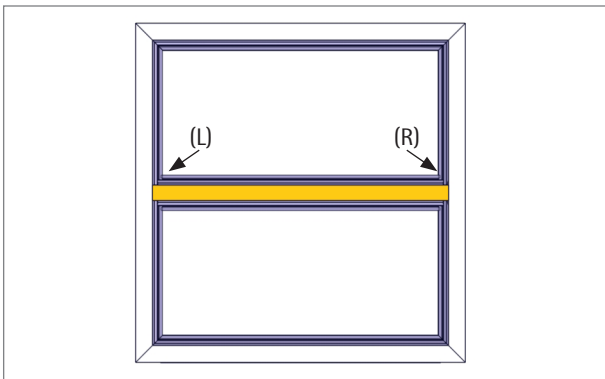
Zusatzarbeiten bei T-Profil als Riegel/Flügelprosse.
