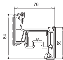
103.381 Verstärkung 113.292, 113.294, 113.295, 113.394
