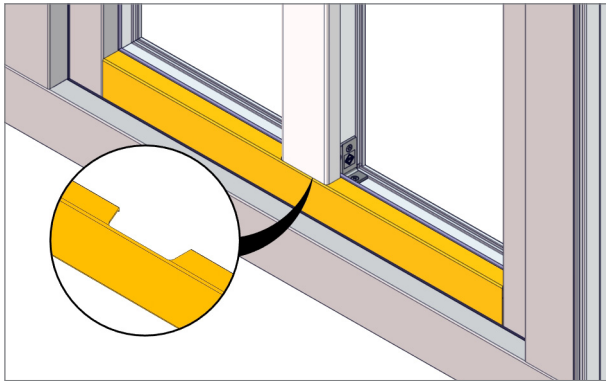
1. Aluminium-Vorsatzblenden vom Flügel im Bereich der Flügelprosse stanzen, siehe Seite 6.48.
