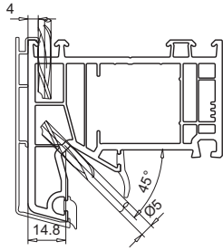
Vorkammerbelüftung Blendrahmen oben
