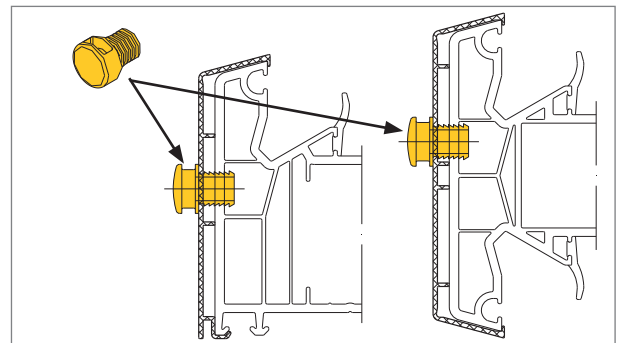
8. Bei Entwässerungsöffnungen, die als Bohrungen \phi 10 mm ausgelegt sind, das Entwässerungsröhrchen 109.225 einsetzen. Für Blendrahmen die Bohrlehre 146.037.1 verwenden.
