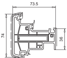
102.358 Verstärkung 113.013
