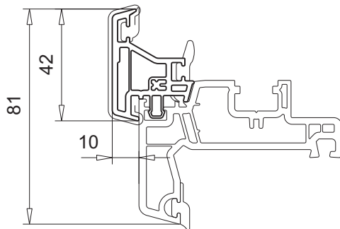
Montagebeispiel mit Flügel 103.389 M.1:2
