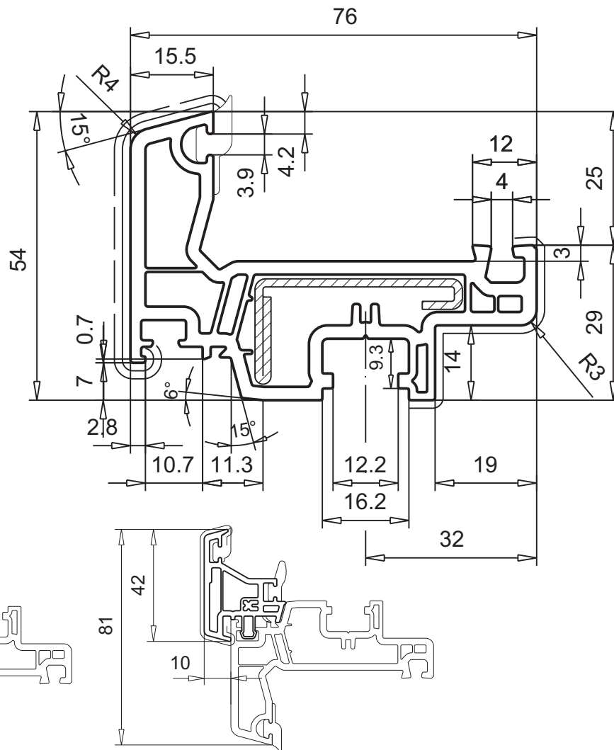
Montagebeispiel mit Stulpprofil 102.308 M.1:2
