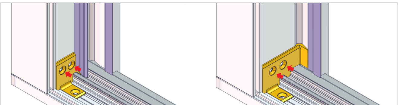
Bohrbild für Falzeckverbinder 106.443 (MD)
