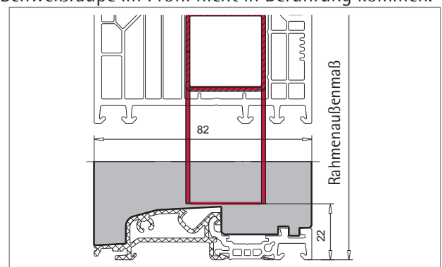
Die Länge der Verstärkungen der Blendrahmen im Schwellenbereich (rot markiert) entspricht dem Rahmenaußenmaß abzüglich mindestens 22 mm
