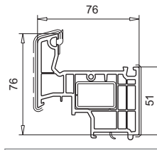
103.384 Aufbauprofil Verstärkung 113.019
