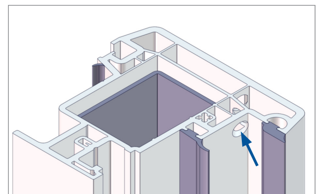
4. Für Stulpprofile in farbiger Ausführung Vorkammern (oben) belüften. bohren ( \phi 5 mm), siehe ab Seite 5.17
