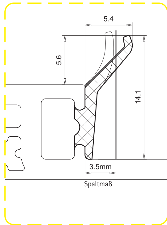
Mitteldichtungen 112.495
