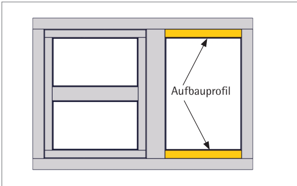
1. a. Aufbauprofil für Fenster 103.384: Fenster vorfertigen inkl. Aluminium-Vorsatzblenden.
