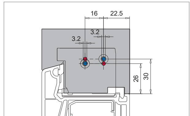
Bohrpositionen ● ● für T-Profil 102.355. Aufgrund der schmalen Verstärkungs-kammer müssen die Bohrpositionen versetzt angebracht werden.
