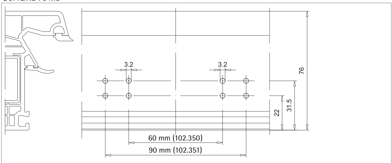
Bohrpositionen ● ● für T-Profil 102.355. Aufgrund der schmalen Verstärkungs-kammer müssen die Bohrpositionen versetzt angebracht werden.
