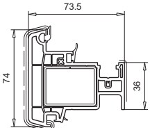
102.356 Verstärkung 113.001
