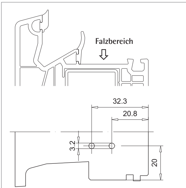
Bohrbild für Falzeckverbinder 106.443 (MD)
