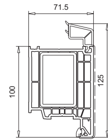
105.403 für flügelüberdeckende Füllungen innen öffnend Verstärkung 113.011, 113.011.5 vorgefräst
