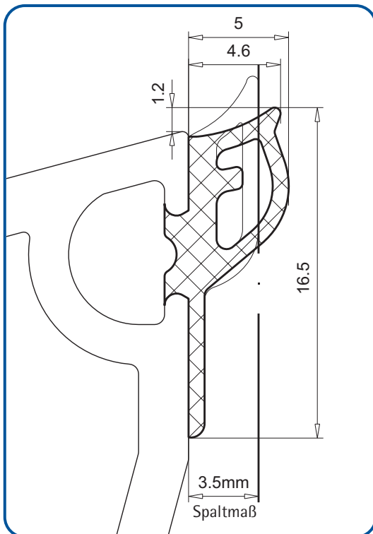
Blendrahmen- und Verglasungsdichtungen 112.493, 112.397 und 112.420
