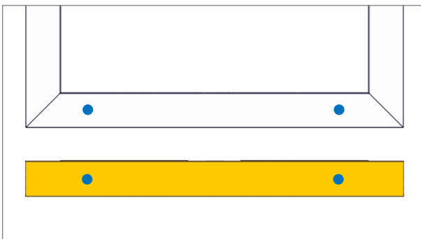
7. Aluminium-Vorsatzblende unten horizontal für Entwässerungsbohrung ( \phi 10 mm) vorbohren. Für Anzahl und Anordnung siehe Seite 5.8.
