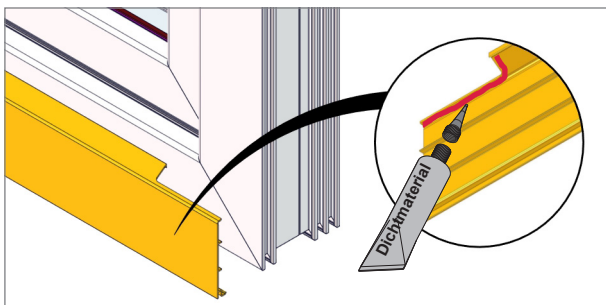
3. Aluminium-Vorsatzblenden unten horizontal im Bereich der Stanzung (L+R) mit geeignetem Dichtmaterial abdichten. Dichtmaterial auf Innenseite anbringen.
