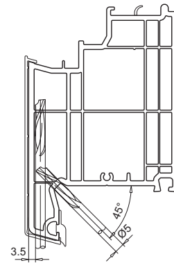
Vorkammerbelüftung Aufbauprofil oben
