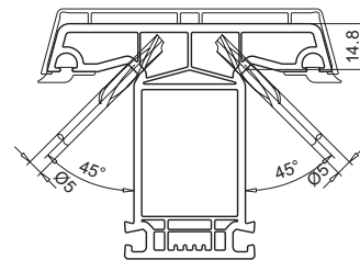
Vorkammerbelüftung Aufbauprofil oben
