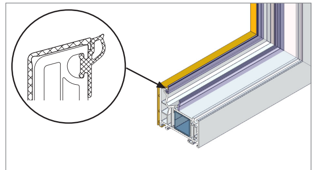
9. b. Bei Festverglasung (MD) Dichtung 112.549 (Handeinzug), bei Festverglasung (AD) werkseitig einextrudierte Dichtung. Für detaillierte Informationen zu Dichtungen siehe ab Seite 6.54.
