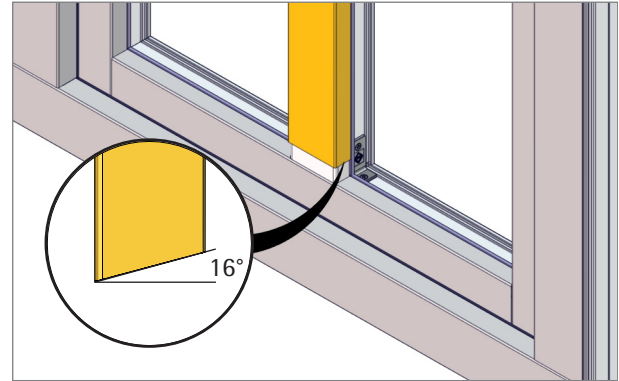
2. Aluminium-Vorsatzblende für Flügelprosse auf Länge schneiden, siehe ab Seite 6.86 und beidseitig die Schnittkanten auf 16° anschrägen.
