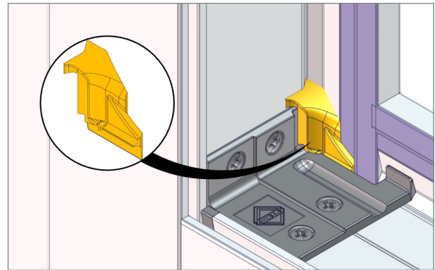
9. Entwässerungshohle zwischen Verbinder und Blendrahmendichtung mit Dichtstopfen 106.395 schließen.
