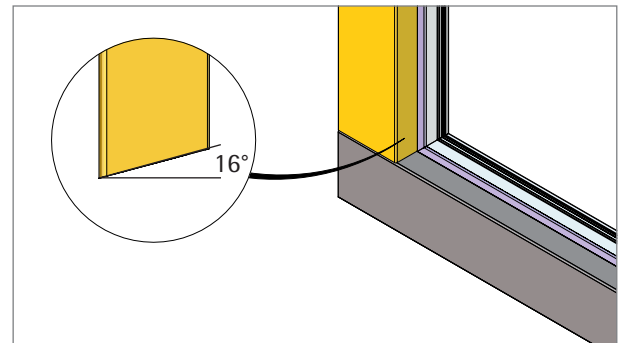
2. Vertikale Aluminium-Vorsatzblende auf Länge schneiden, siehe ab Seite 6.86. Beidseitig die Schnittkanten auf 16° anschrägen.
