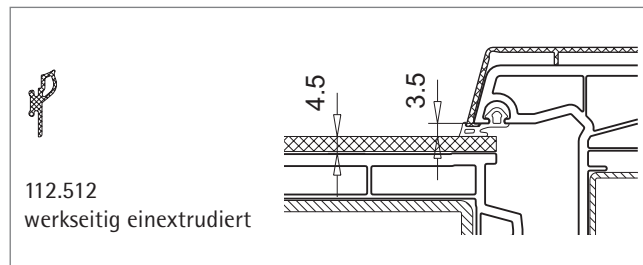
Variante 2: Sonderausführung mit Aluminium-Vorsatzblende, Spaltmaß 3,5 mm, Dichtung durch Handeinzug
