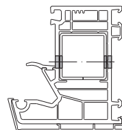
Dübellochbohrung dübelabhängig
