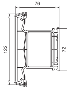
102.357 Verstärkung 113.011
