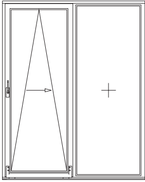
zweiteilige Abstelltür Schema: A Kipp-Schiebe/Fest
