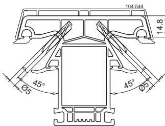
Vorkammerbelüftung Stulpprofile oben
