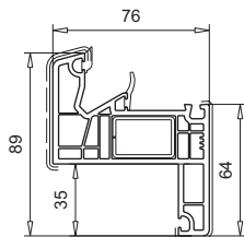
101.358 Verstärkung 113.019
