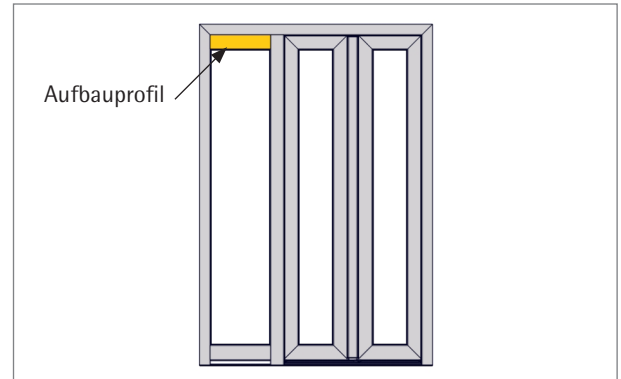
1. b. Aufbauprofil für Haustür 105.402: Türelement vorfertigen inkl. Aluminium-Vorsatzblenden.
