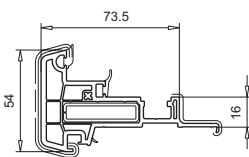
102.354 Verstärkung 113.028
