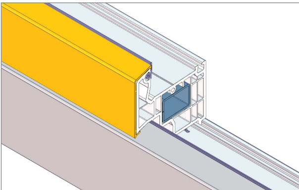
7. Aluminium-Vorsatzblende auf Aufbauprofil klipsen.
