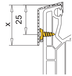
Montagebeispiel für gekürzte Aluminium-Vorsatzblenden
