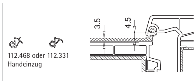
Variante 3: Sonderausführung, Spaltmaß 4,5 mm, Dichtung durch Handeinzug
