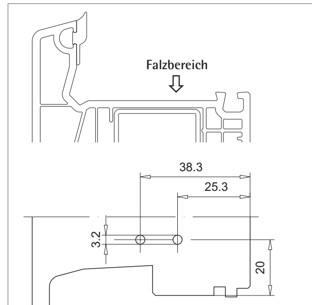
Bohrbild für Falzeckverbinder 106.442 (AD)
