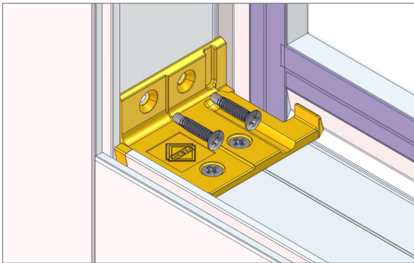
8. Verbinder am Blendrahmen mit 2 Schrauben M3,9 x 19 mm (141.003.019.000) verschrauben.
