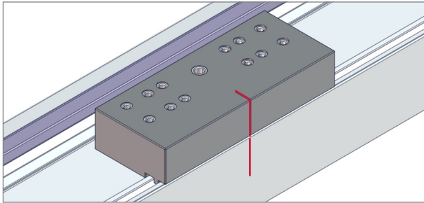
Bohrschablone 146.032.0 (AD), Mittelachse rot markiert
