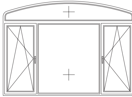
✓ ◆ Korbbogenfenster Dreh-Kipp/Fest/Dreh-Kipp
