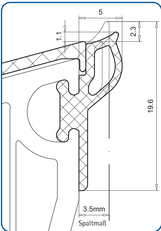
Verglasungsdichtung 112.512, 112.549 und 112.485
