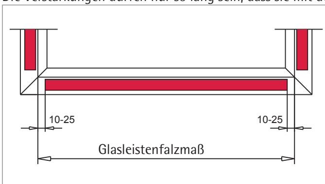
Die Länge der Verstärkungen (rot markiert) entspricht dem Glasleistenfalzmaß abzüglich 20 bis 50 mm
