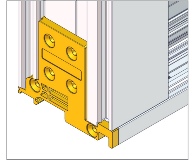
Montagebeispiel
