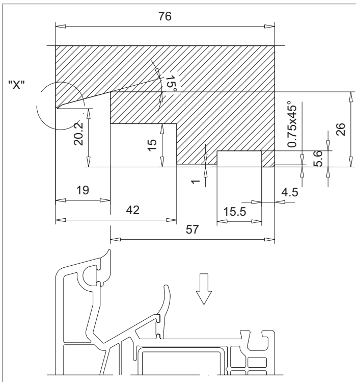
Fräszzeichnung für die Werkzeugbestellung MD
