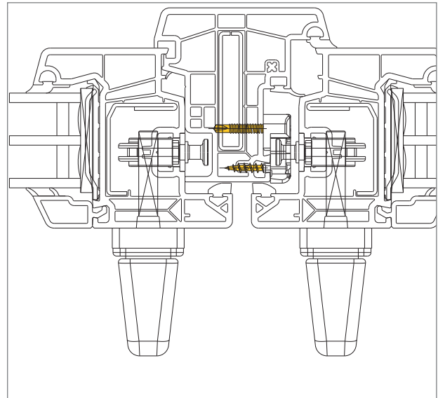
Stulpprofil 102.358 mit 2 Griffoliven
