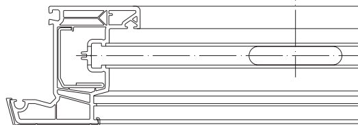
Schlosskastenbohrung/-fräsung beschlagabhängig
