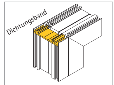
Montagebeispiel
