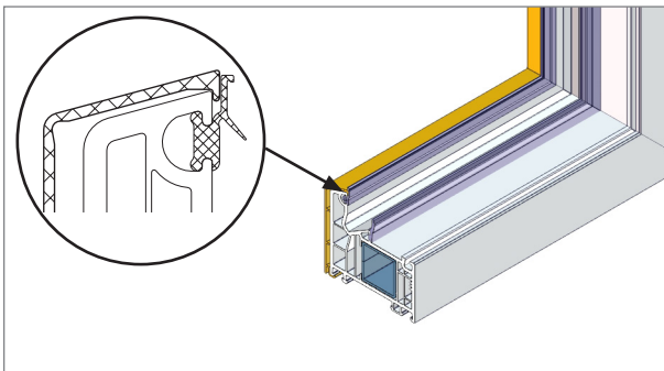
9. a. Anschlagdichtung werkseitig einextrudiert. Für detaillierte Informationen zu Dichtungen siehe ab Seite 6.54.
